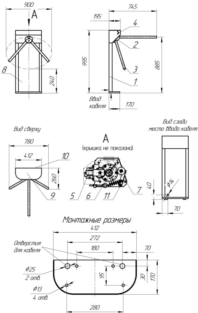
Габаритные и установочные размеры турникетов серии «Ростов-Дон Т83М1»
